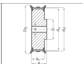
Zeichnungsteile
